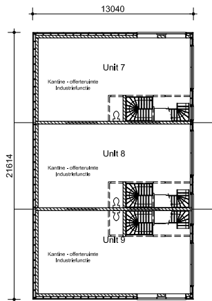
eerste verdieping
