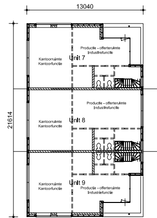
tweede verdieping
